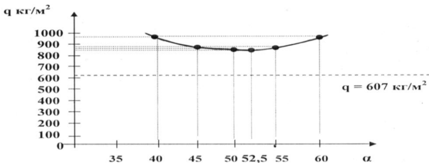
Рис. 2. График «Q – \alpha » для определения минимальную несущую способность Q_{min} при угла \alpha = 52,5^\circ
