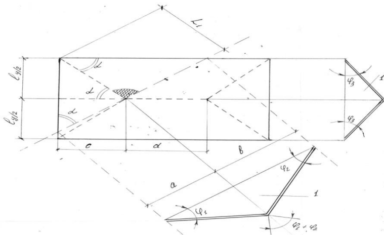
Рис. 1. Расчетная модель сборных железобетонных плит перекрытий опертых по контуру
