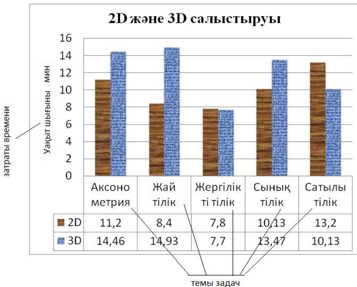
Рисунок 3 – Сравнение затрат времени на выполнение чертежей в 3D-формате и 2D-формате
